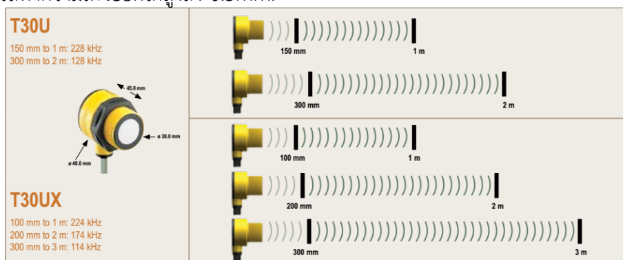
รูปที่ 2 ตัวอย่างอัลตราโซนิกเซ็นเซอร์แบบความถี่สูง
