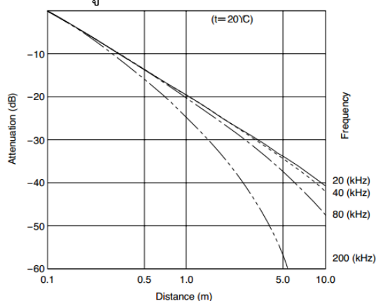
รูปที่ 1 การลดทอนคลื่นอัลตราโซนิกในแต่ละความถี่
